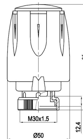
Рис. 2. Габаритные размеры, мм.
