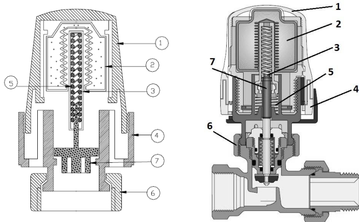
Рис 1. Основные элементы конструкции.
