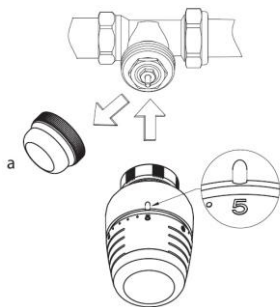
Рис 4.а Установка термостатической головки.
