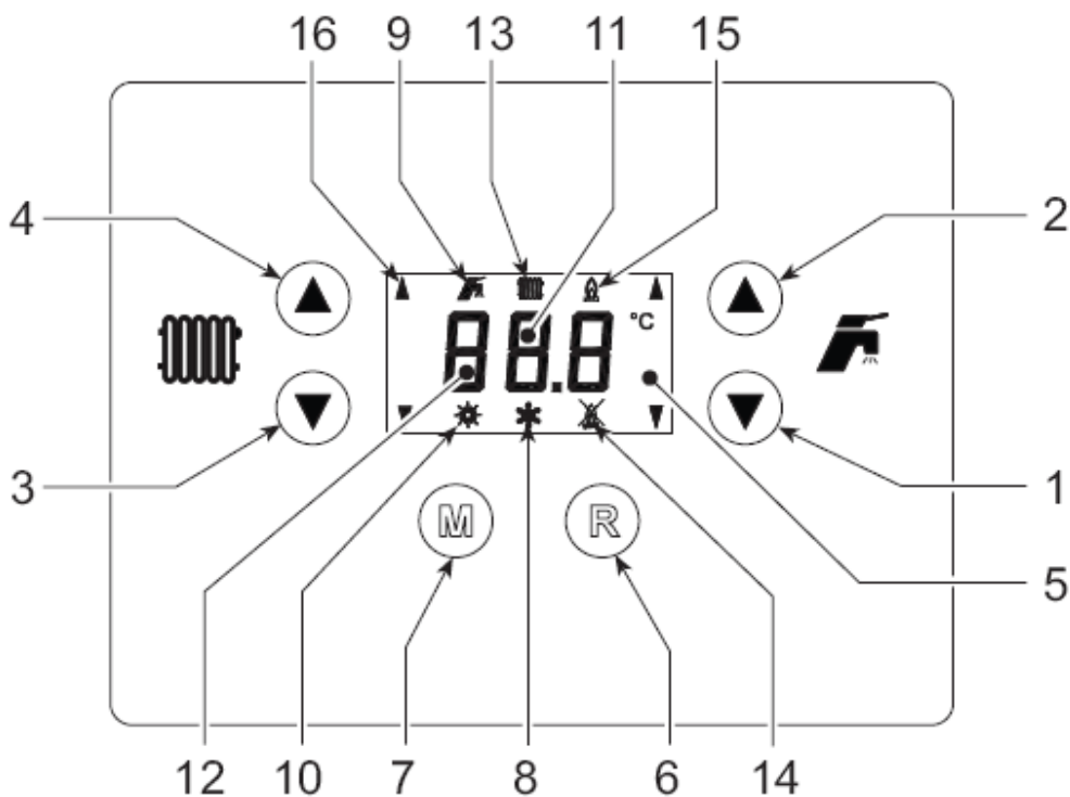
Рис. 1 - Панель управления
