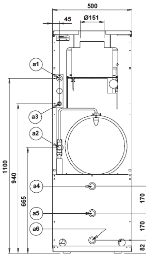
Рис. 17 – Схема подключения
