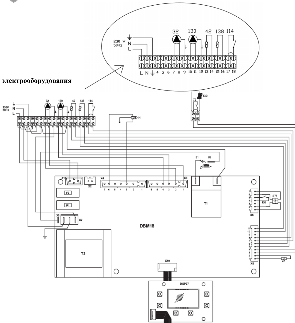
Рис. 26 – Схема электрооборудования
