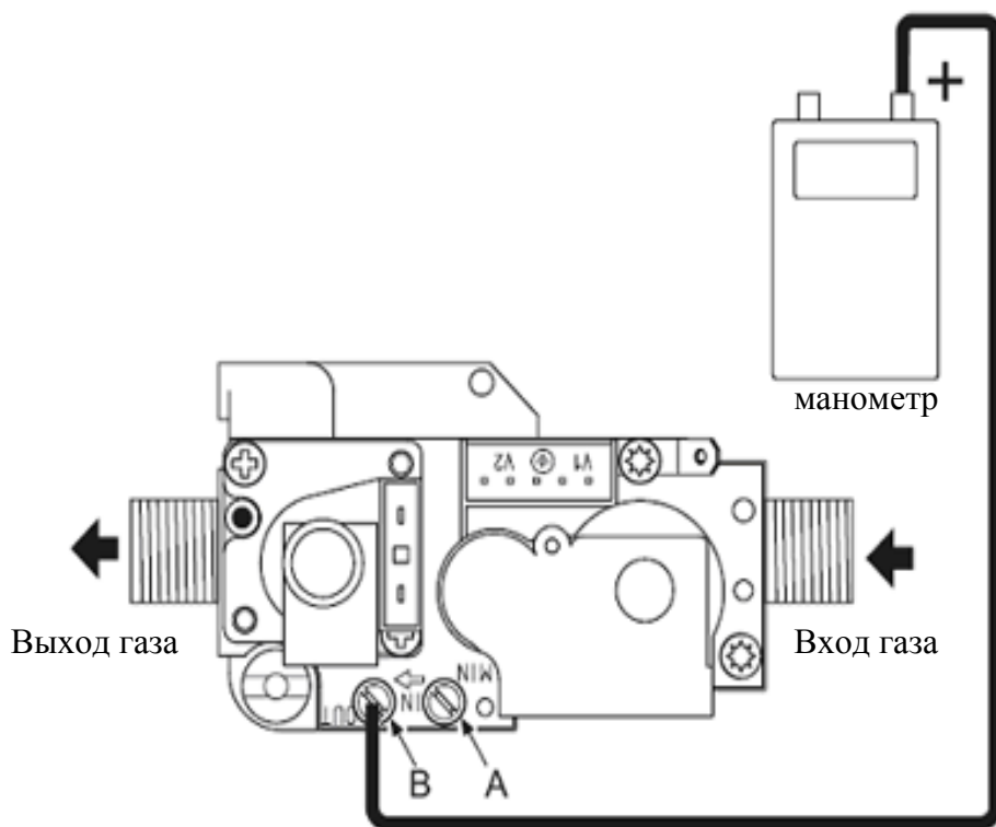
Рис. 19 газовый клапан
