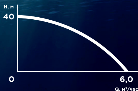
График рабочей характеристики
